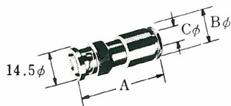
1図 BNC-P-HV
