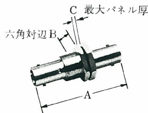
1図 BNC-BA-JJ-HV
