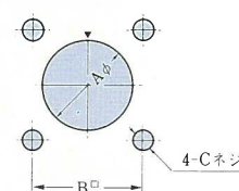
取付寸法
